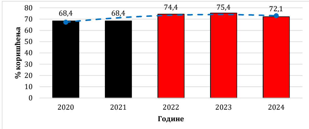
Дијаграм бр. 3.5.1. Тренд % употребе заштитних система (укупно возачи, сувозачи, путници и деца) у путничким аутомобилима и доставним возилима до 3,5t у полицијској управи Пријепоље (2020-2024)
