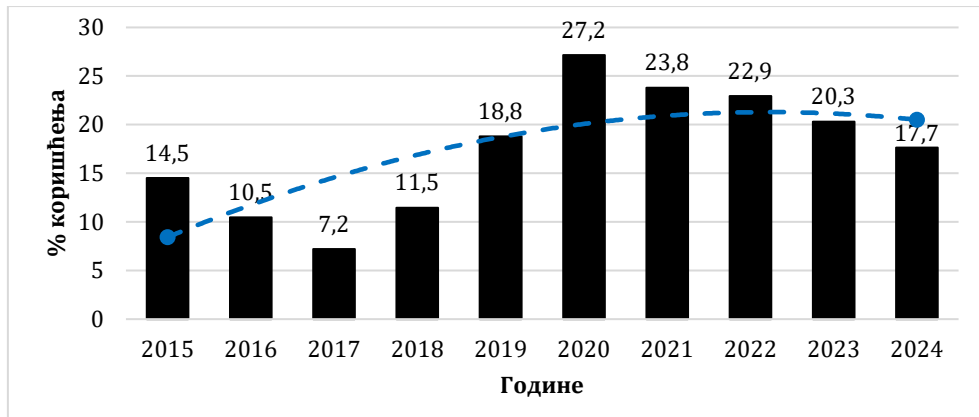
Дијаграм бр. 3.3.1. Тренд % употребе сигурносног појаса на задњем седишту у путничким аутомобилима и доставним возилима до 3,5t у полицијској управи Шабац (2015-2024)
