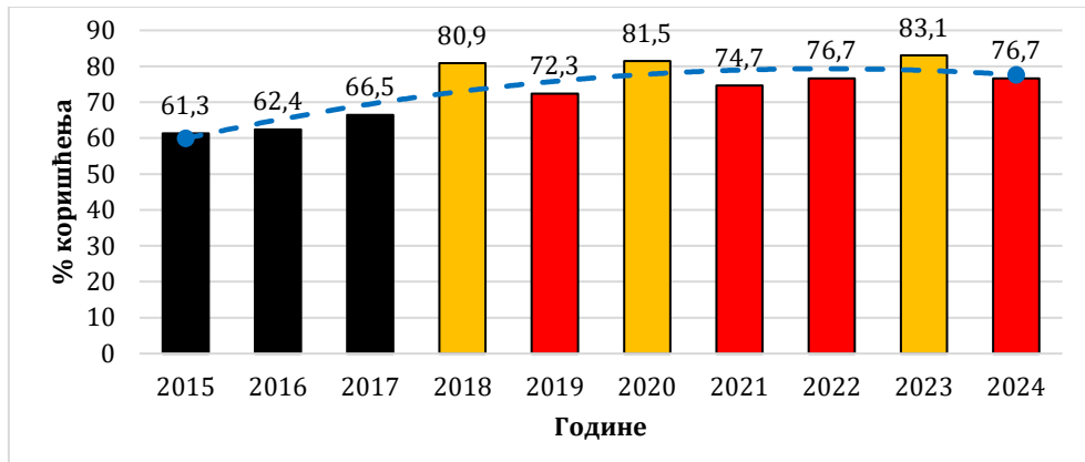
Дијаграм бр. 3.2.1. Тренд % употребе сигурносног појаса на предњем седишту у путничким аутомобилима и доставним возилима до 3,5t у полицијској управи Шабац (2015-2024)
